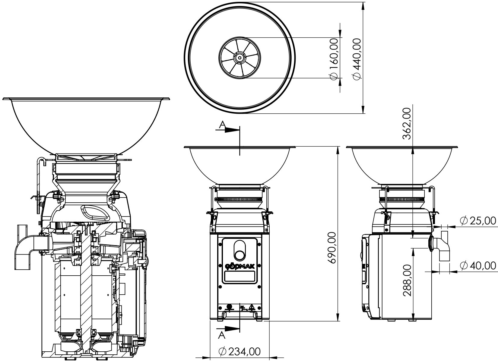
KESİT A-A ÖLÇEK 1 : 6
